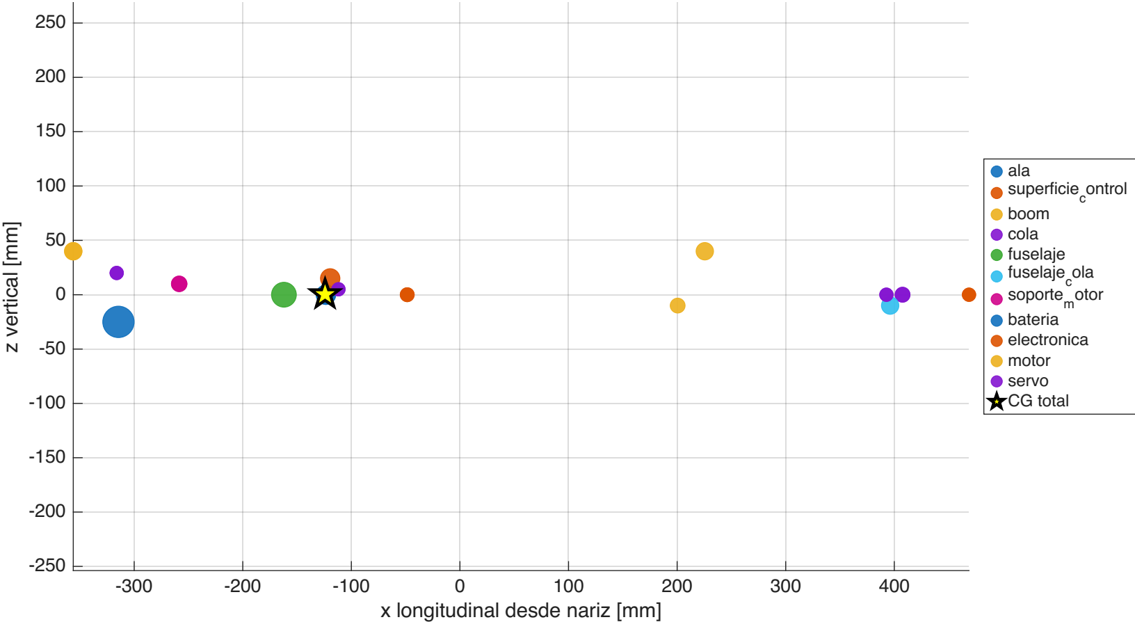
Distribucion de masa y CG - vista lateral
